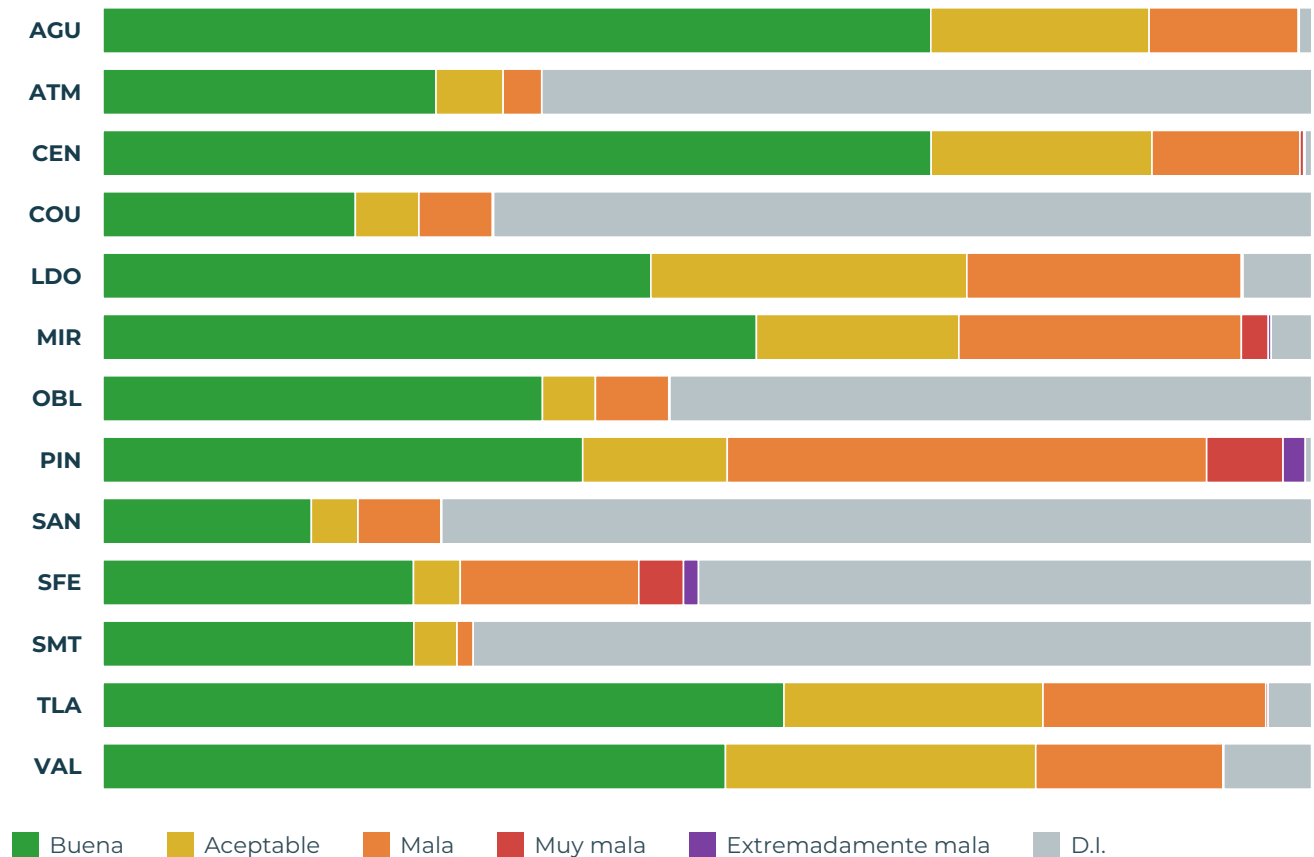
Figura 3. Horas del año según categoría de calidad del aire, por estación.
